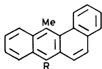
(5) R = Me (7) R = CH 2
